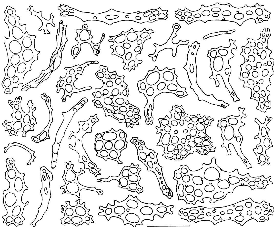
Рис. 5. Спикулы шупалец.
